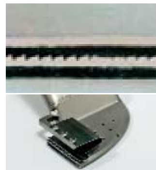
При сварке пленок ТРО благодаря запатентованной насадке с прихватом осуществляется предварительная зачистка пленки. (принадлежность)
