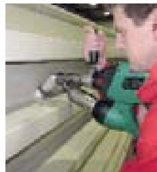
Угловая насадка 45° для WELDPLAST S2 облегчает сварку в труднодоступных местах (принадлежность).
