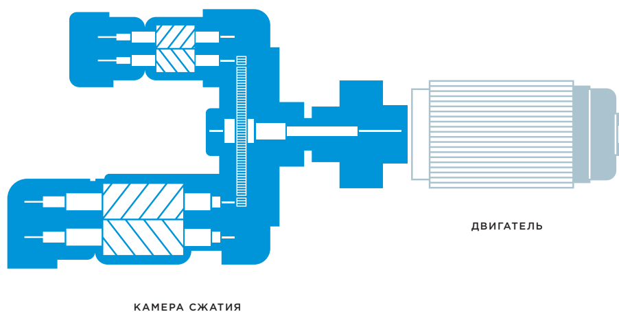
КАМЕРА СЖАТИЯ
